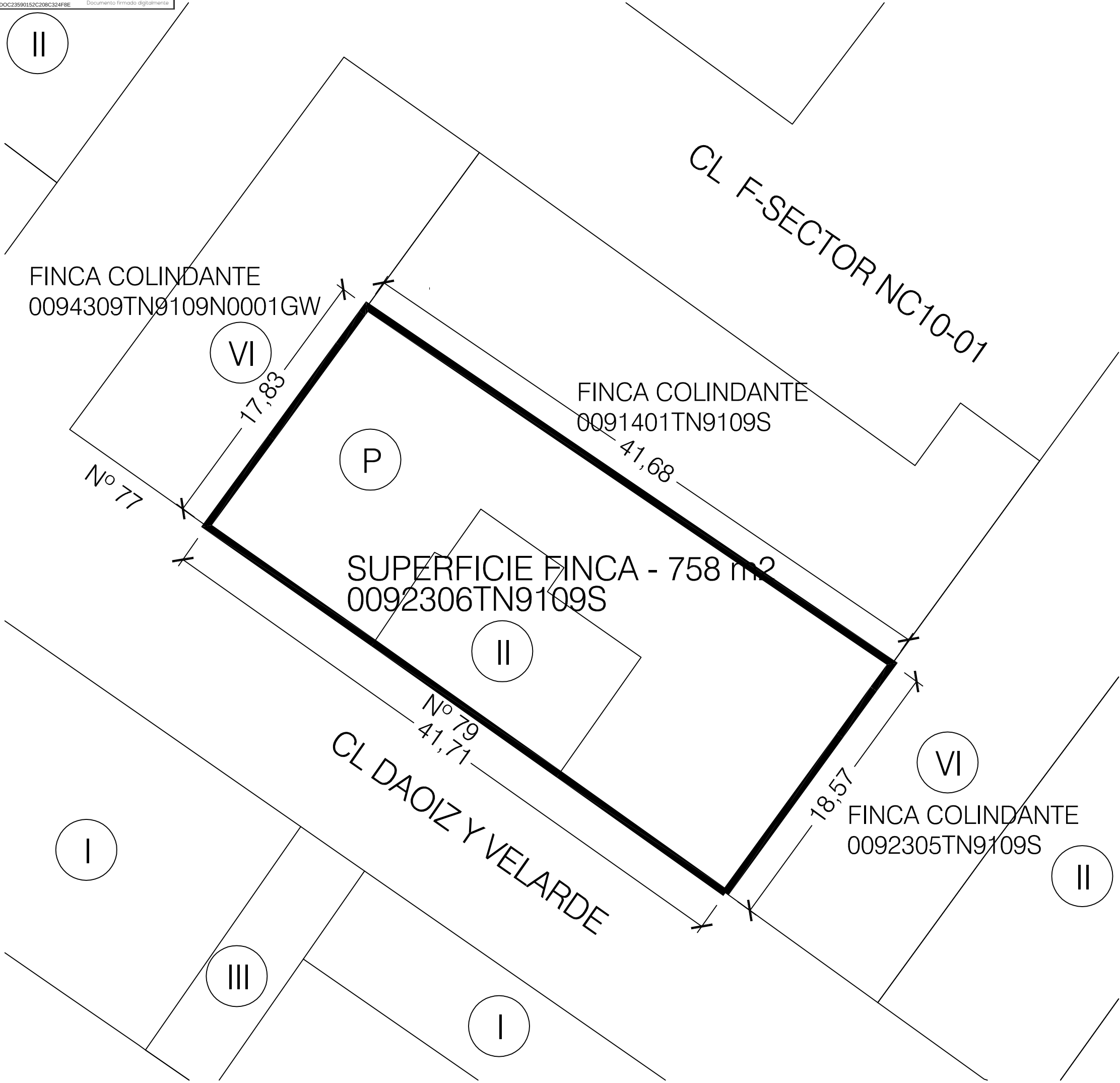
SITUACIÓN. ESC 1/2000 PARCELA. ESC 1/250
