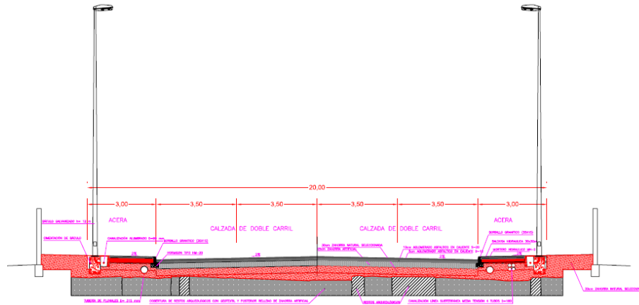
SECCIÓN TRANSVERSAL TIPO
