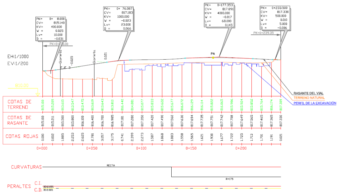
PERFIL LONGITUDINAL EJE 1
